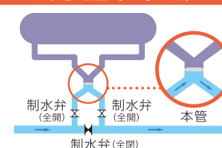
緊急遮断時の水の流れ
