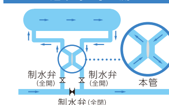
通常時の水の流れ
